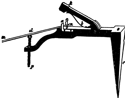
Fig. 115.—Barth's setting-iron.
